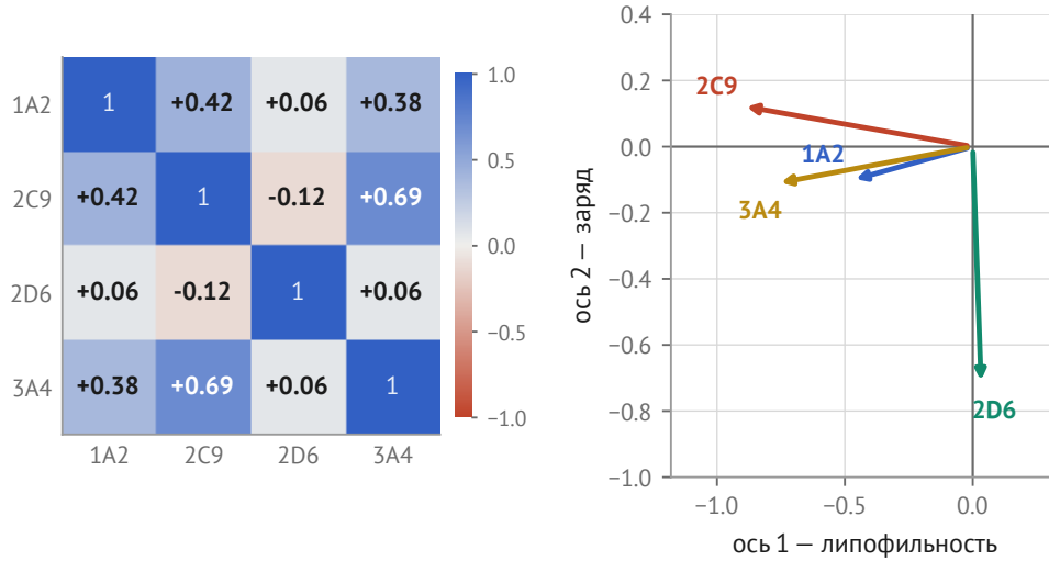
Рис. 7. Слева — ранговая корреляция \rho IC_{50} между ферментами, посчитанная по общим соединениям (от 230 пар у 2C9–2D6 до 473 у 2C9–3A4). Справа — нагрузки факторной модели ранга 2 на те же данные: каждая стрелка показывает, насколько фермент участвует в каждой из двух общих осей. Первая ось нагружает 2C9, 3A4 и слабее 1A2, на 2D6 стоит на нуле; вторая ось — почти исключительно 2D6.
